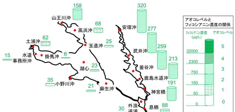
R5年8月3日にアオコ情報で発表された地点ごとのフィコシアニン濃度(µg/L)
