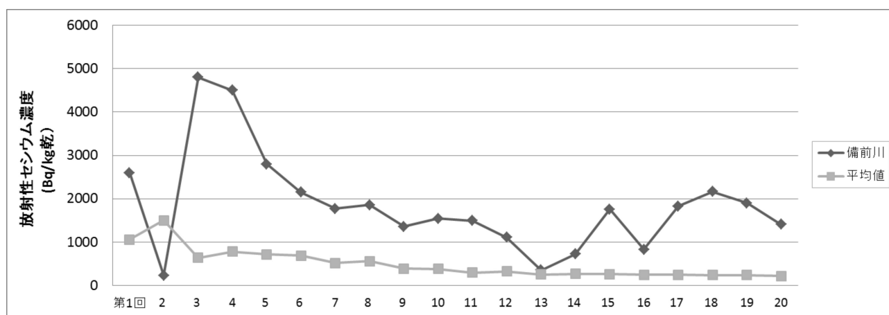
第20回調査において放射性セシウム濃度の高い地点の数値の推移 (セシウム134+セシウム137)
