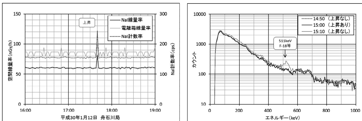
図1 RI (F-18 と推定) 投与者接近による空間線量率 (2分値) の上昇例 左:トレンドグラフ 右:MCA スペクトルグラフ (舟石川局:平成30年1月12日)
