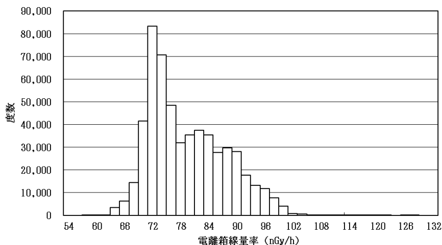
図2 空間線量率度数分布 (電離箱線量率)
