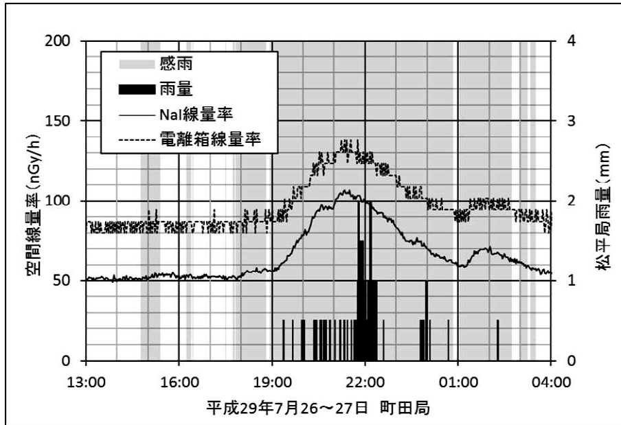
図 4 空間線量率 (2 分値) の上昇
