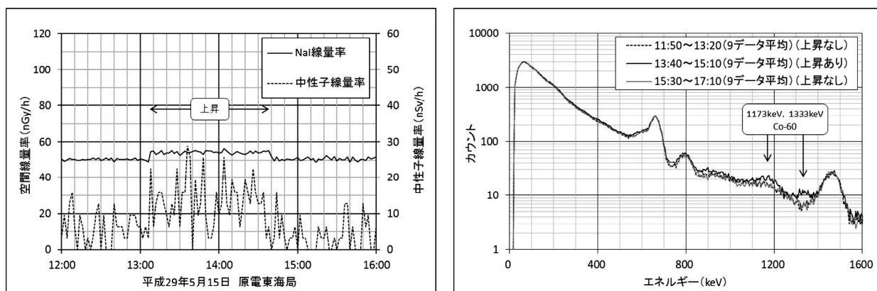
図2 Co-60 \gamma 線源及び中性子線源による空間線量率及び中性子線量率 (2分値) の上昇例 (Co-60 と Cf-252 を利用した密度水分計を周辺道路工事で使用したと推定) 左:トレンドグラフ 右:MCA スペクトルグラフ (トレンドグラフに対し, 10~20分程度遅れ) (原電東海局:平成29年5月15日)
