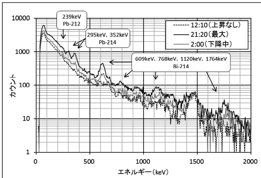
図 5 町田局の MCA スペクトルグラフ
