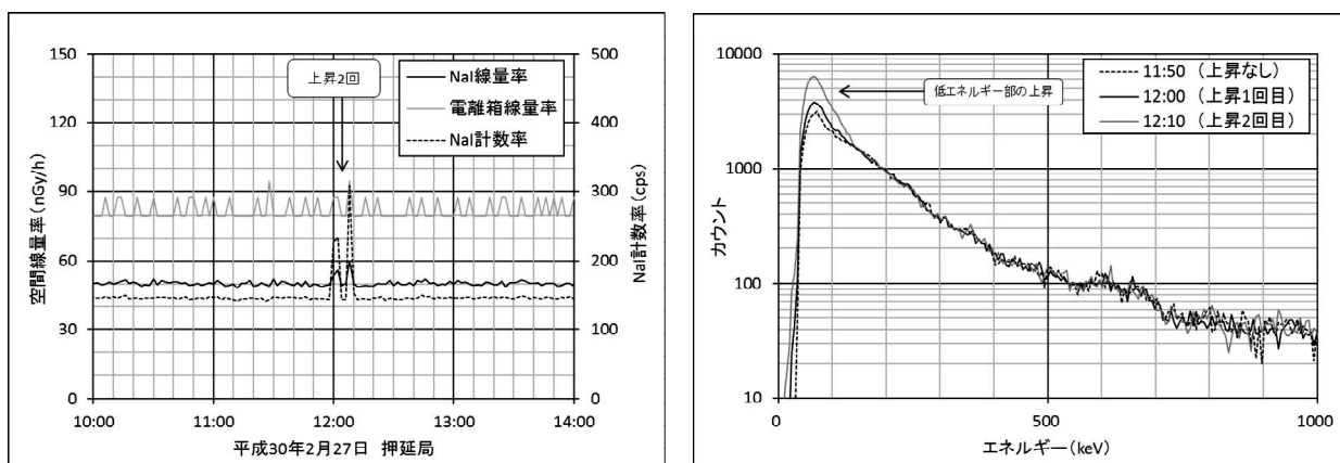
図3 ガス配管管理工事のX線非破壊検査による空間線量率 (2分値) の上昇例 左:トレンドグラフ 右:MCA スペクトルグラフ (押延局:平成30年2月27日)
