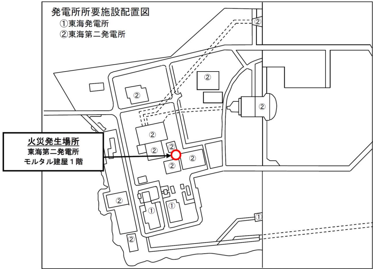
東海・東海第二発電所 施設配置図
