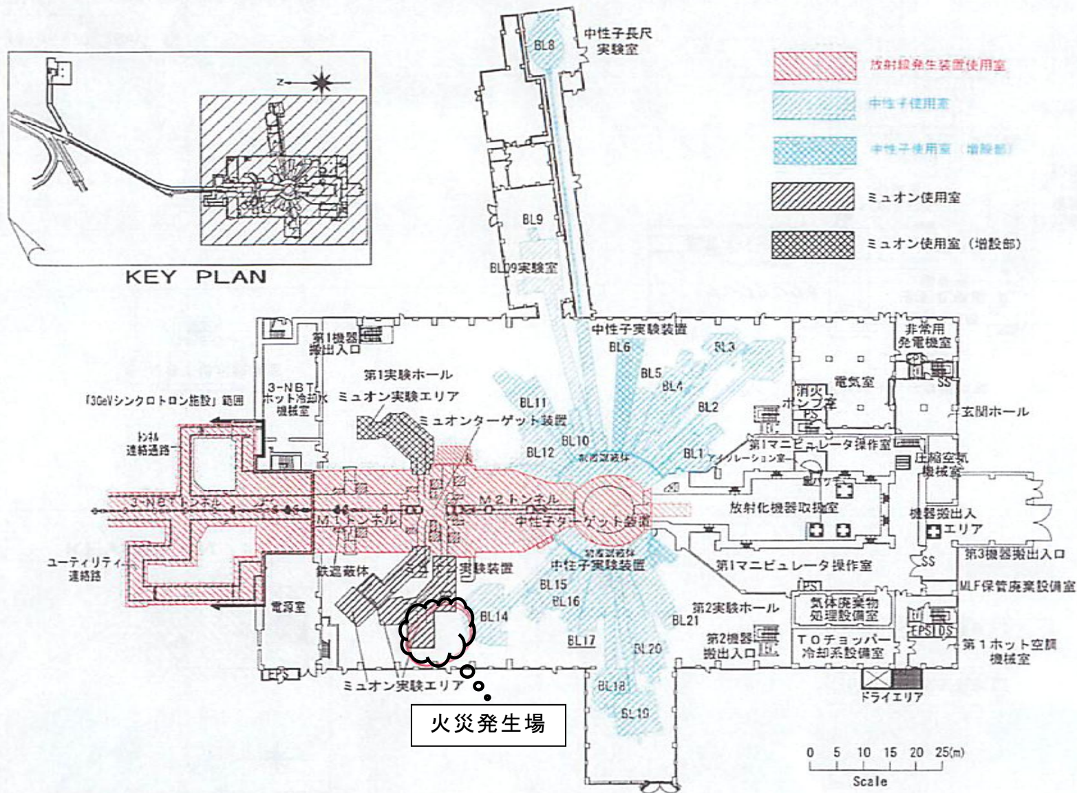
図2 物質・生命科学実験施設 1階平面図
