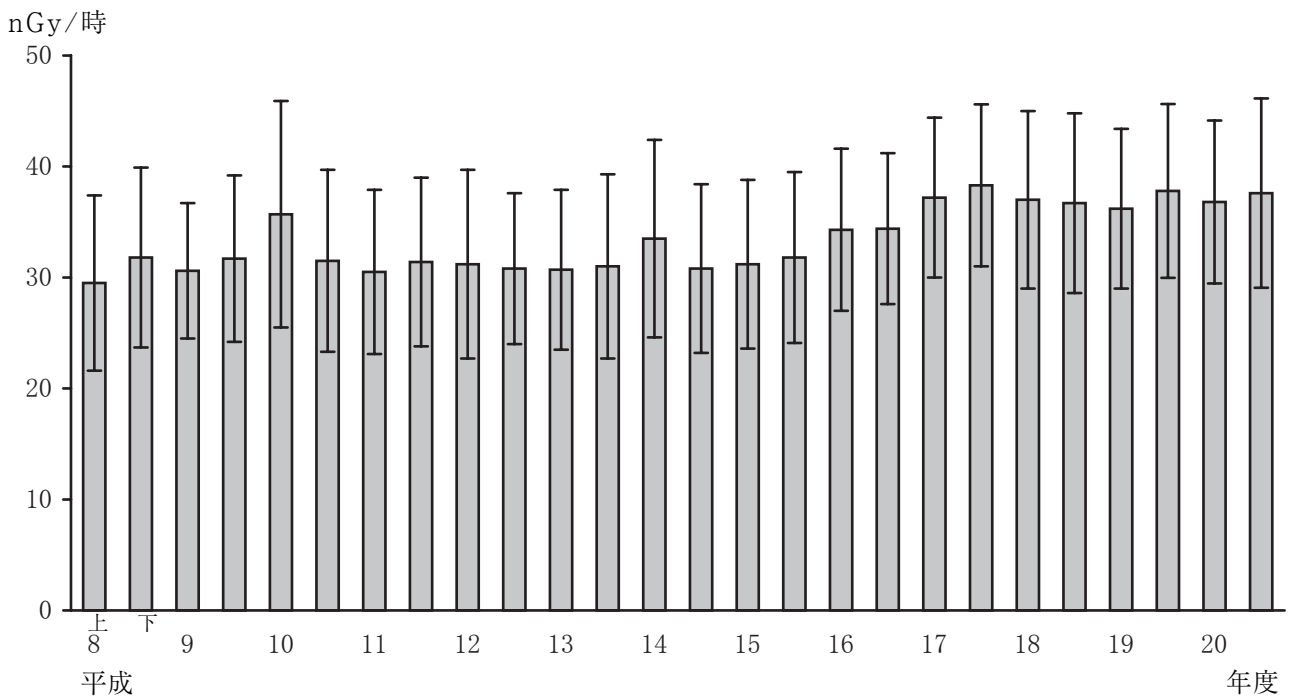
空間γ線量率（サーベイ）経年変化
