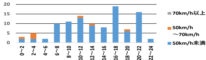
国道6号における時間別・危険認知速度別 人身事故の発生状況（過去3年）
