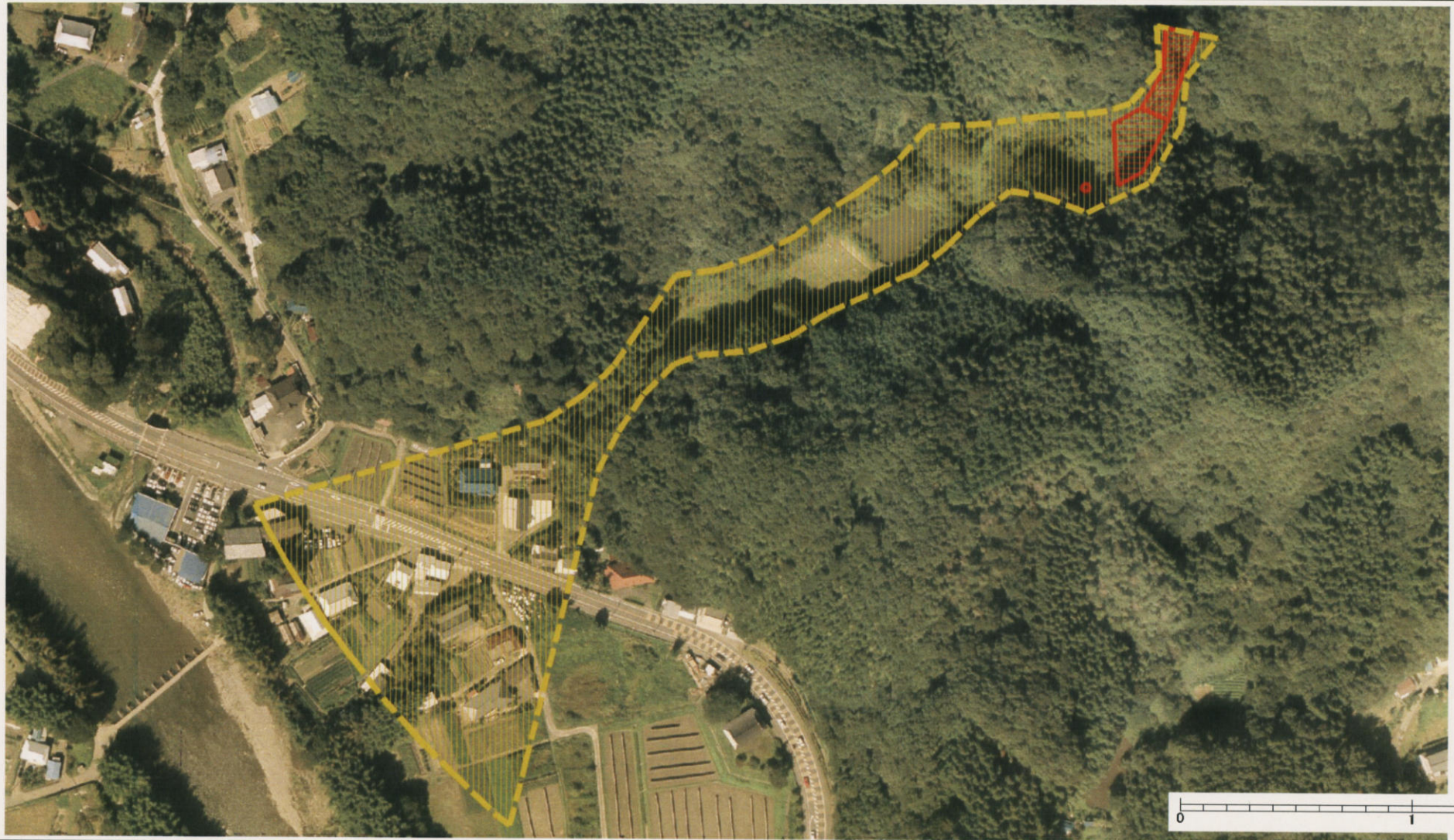
様式-3 (土) 土砂災害警戒区域・土砂災害特別警戒区域 区分図 (その2)
