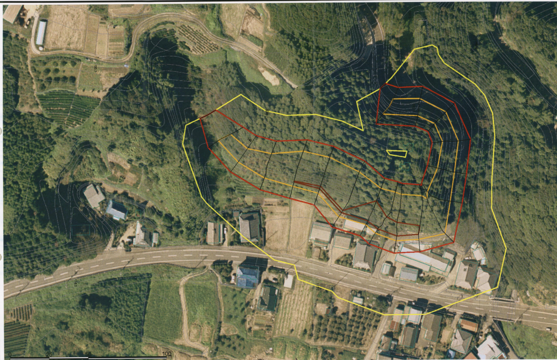
様式-3(急) 土砂災害警戒区域・土砂災害特別警戒区域 区域図(その2)
