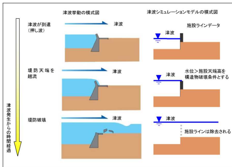
図-3-3.津波越流時破壊の模式図
