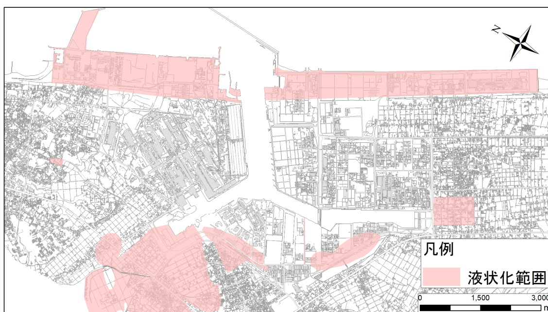
図-5-2.鹿島港における液状化範囲
