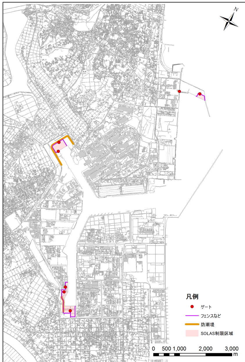
図-2-9.鹿島港の SOLAS 制限区域・防潮堤及びフェンス・ゲートの位置(民間バースを除く)
