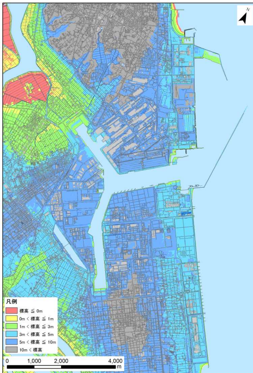
図-2-4.鹿島港の標高図（現況地形）
