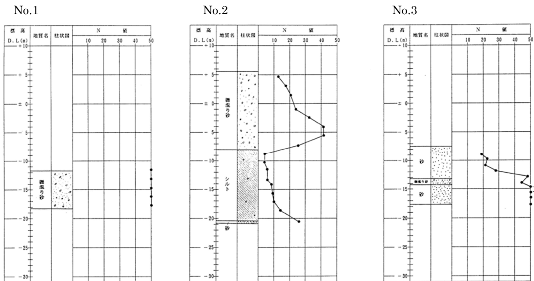
図-2-6. ボーリング柱状図 鹿島港湾計画（H19.3）などより抜粋
